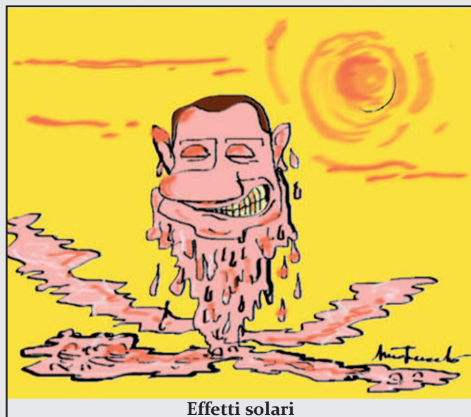
Effetti solari
